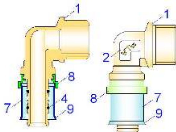
Рис.3.3.2.р.2. Пресс-фитинг
