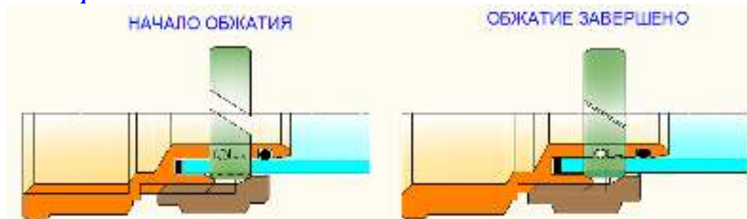
Рис.3.4.п.2. Стадии обжатия МПТ
