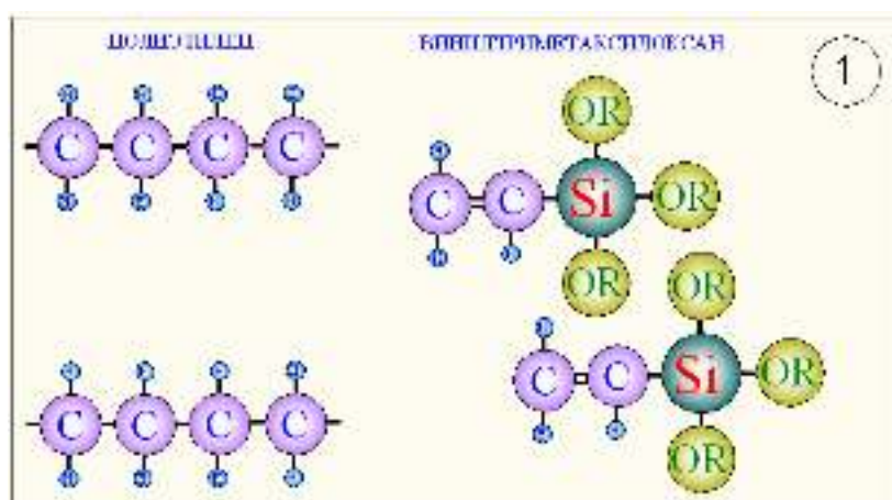
Рис.2.2.п.3 Этапы сшивки полиэтилена по методу В
