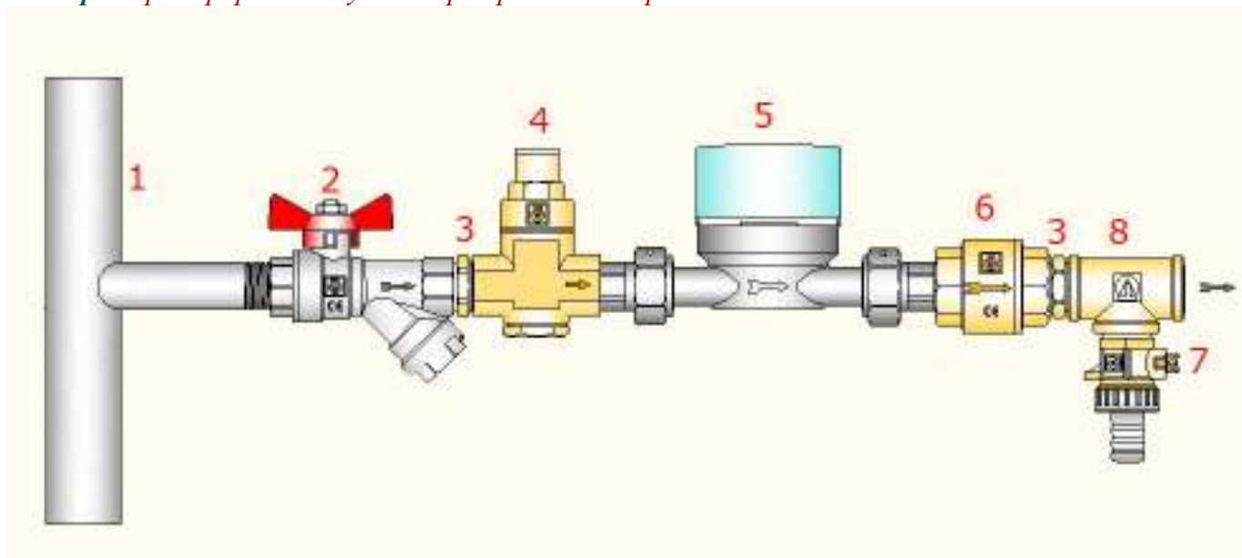
Рис.5.1.p.1 Пример решения узла квартирного водопроводного ввода
