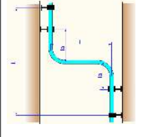
Z-образный компенсатор
