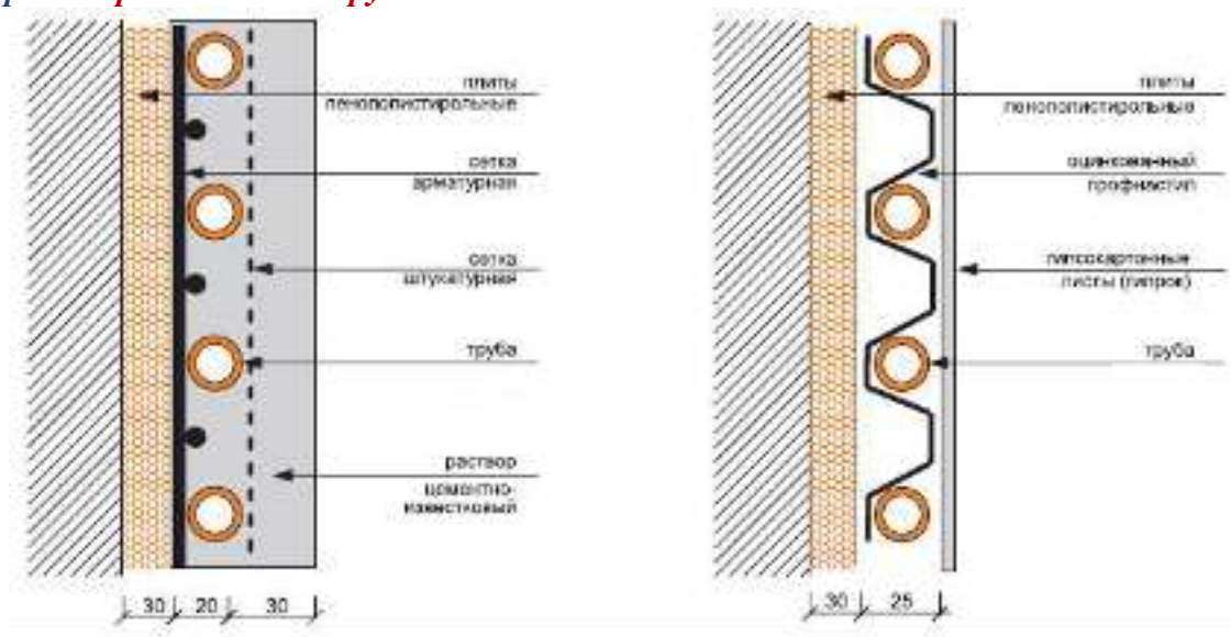
Рис.5.4.р.6 Варианты конструктивного исполнения теплых стен
