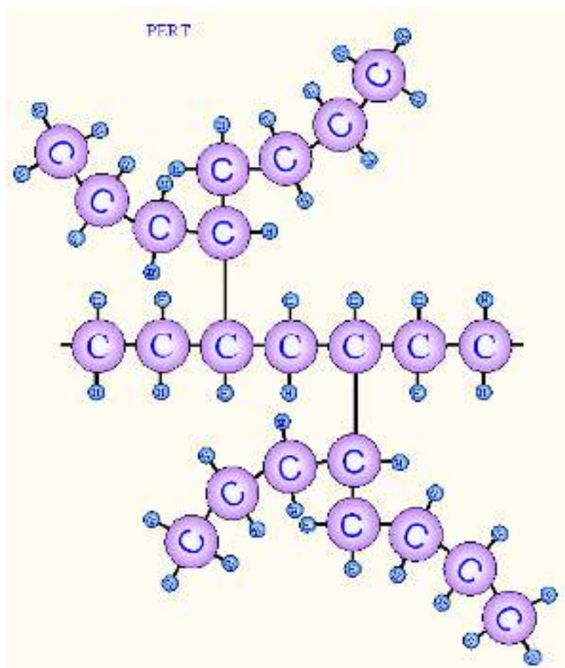
Рис.2.1.р.10 Химическая структура PERT
