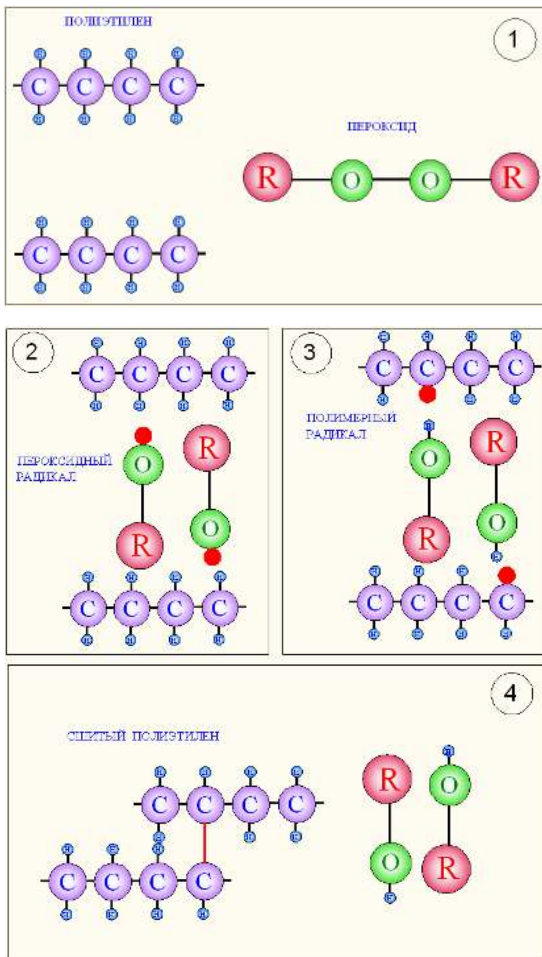
Рис.2.2.р.2 Этапы шивки полиэтилена по методу А
