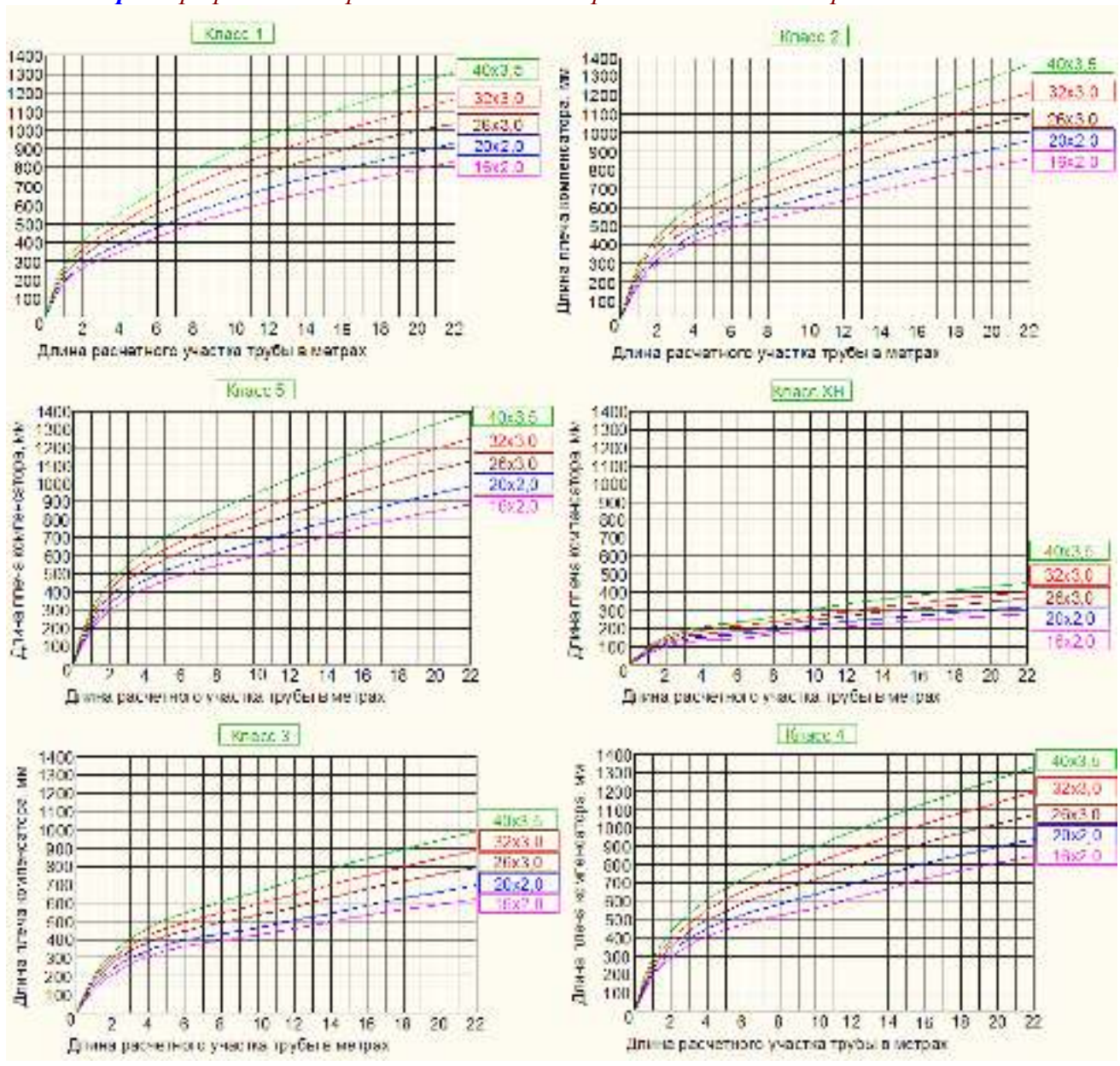
Рис.4.2.4.р.8 Графики для определения плеча Г-образного компенсатора
