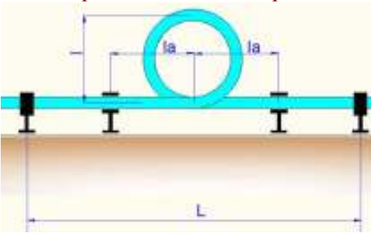
Петлеобразный компенсатор
