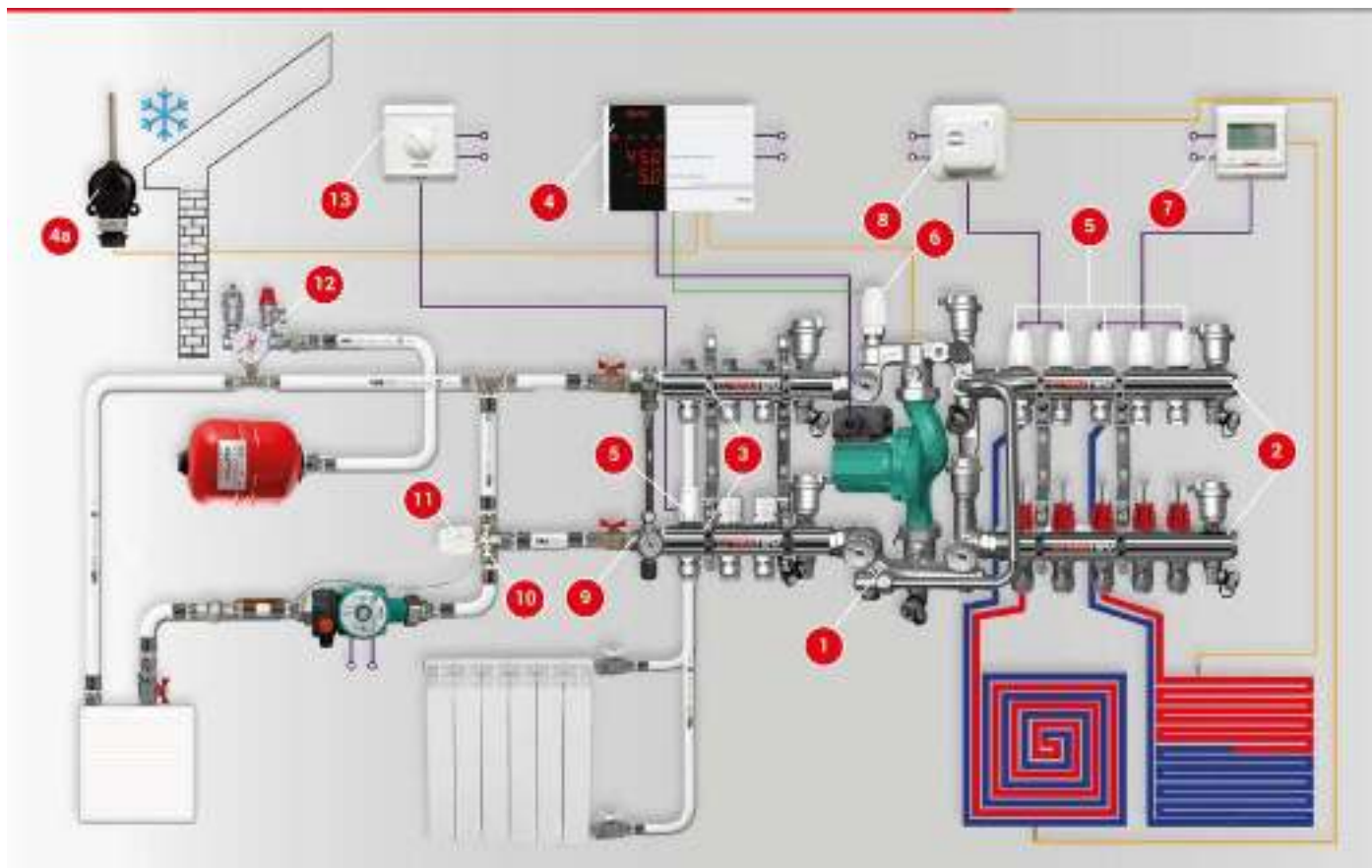
Рис.5.3.1.13 р.3 Комбинированная система отопления с автоматическим управлением
